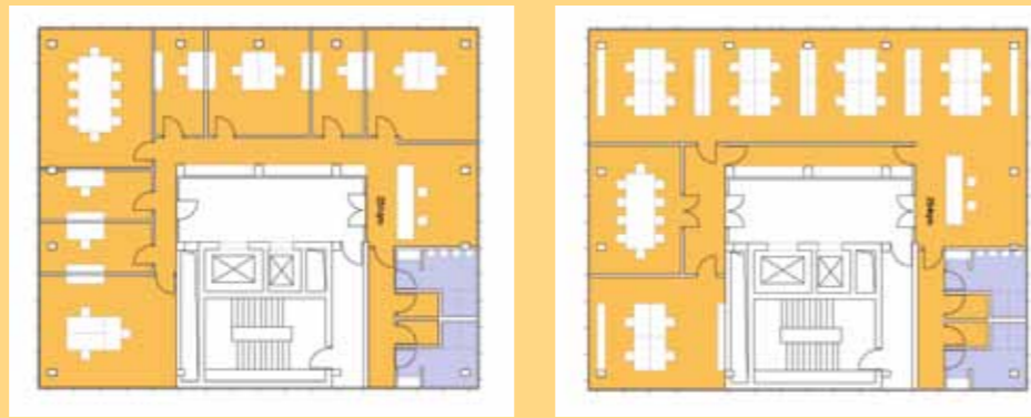
Rund 250 Quadratmeter Fläche hat eine Büro-Etage im Katharinenturm. Die Flächen können entweder für die Nutzung eines großen Büros oder durch Trennungen zu mehreren Arbeitsräumen unterschiedlicher Größe ausgestaltet werden.
